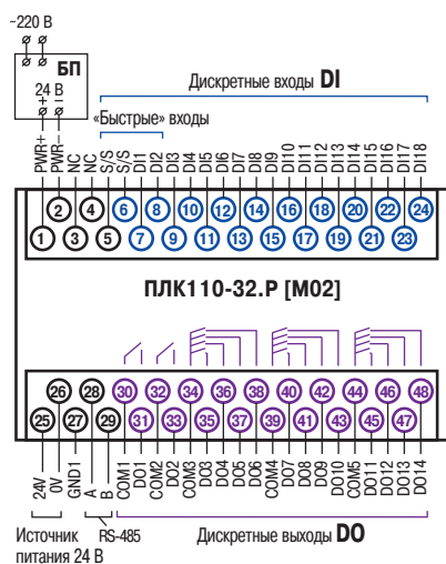
Схема расположения и назначение клемм ПЛК110-24.32.Р [M02]
