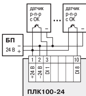
ПЛК100-24, датчик p-n-p-типа
