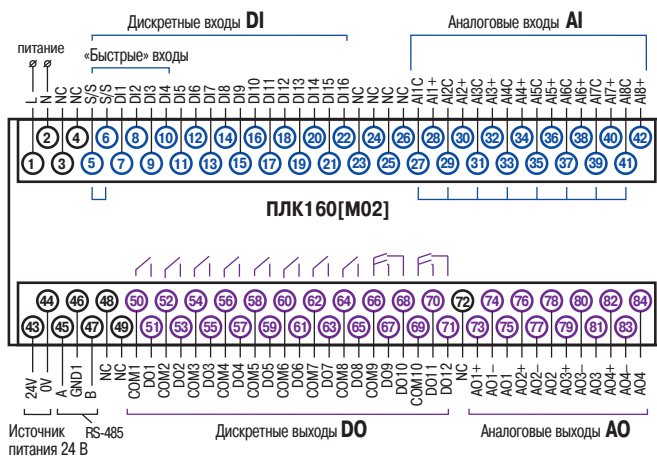
Схема расположения и назначение клемм ПЛК160[M02]
