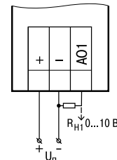
Схема подключения к аналоговому выходу нагрузки в виде напряжения
