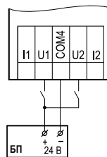
Схема подключения к универсальным входам, работающим в дискретном режиме датчиков типа «сухой» контакт
