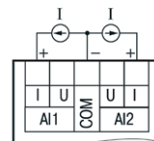
Подключение датчиков с токовым выходом
