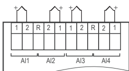
Подключение терморезисторов
