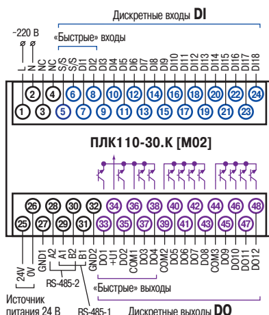
Схема расположения и назначение клемм ПЛК110-220.30.К [M02]
