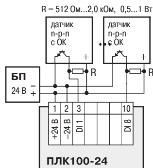
ПЛК100-24, датчик n-p-n-типа
