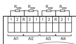
Подключение термометров сопротивления
