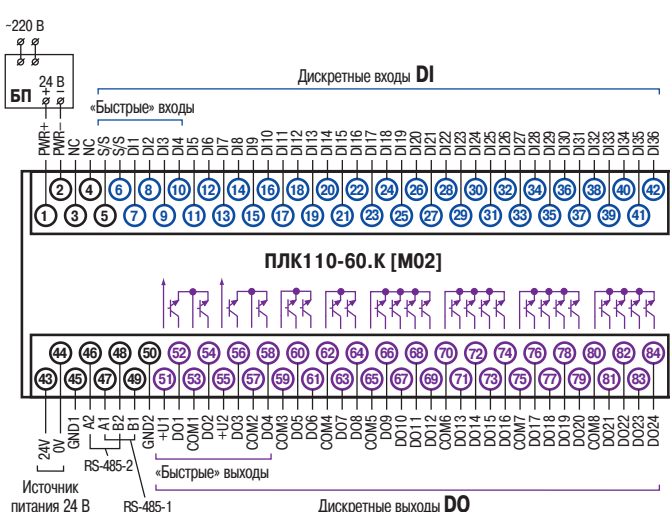
Схема расположения и назначение клемм ПЛК110-24.60.К [M02]
