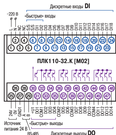
Схема расположения и назначение клемм ПЛК110-220.32.К [M02]
