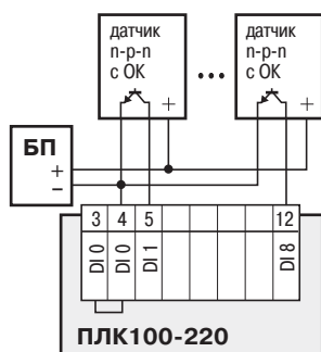
ПЛК100-220, датчик n-p-n-типа
