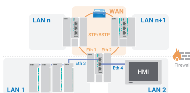
Схема 2. Порты Ethernet 1 и Ethernet 2 объединены в мостовое подключение к глобальной сети (WAN), защищенное межсетевым экраном. Порты Ethernet 3 и Ethernet 4 являются отдельными изолированными сетевыми интерфейсами для подключения к локальным сетям (LAN).
