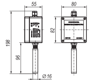
Настенное исполнение H4
