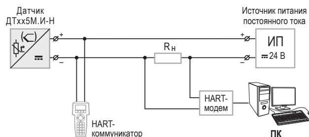
Схема передачи цифрового сигнала от датчика к устройству, поддерживающему HART-протокол
