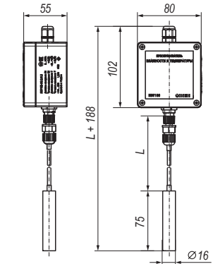
Настенное исполнение H4
