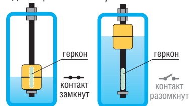
ПДУ с нормально-замкнутым контактом
