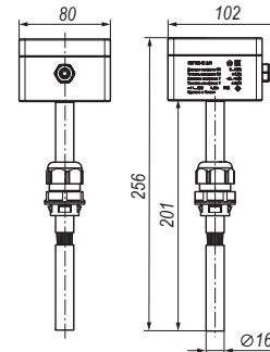
Канальное исполнение K1
