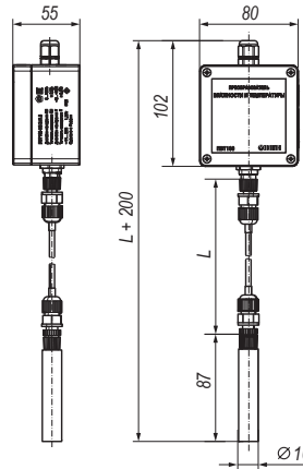
Настенное исполнение H5 с выносным зондом
