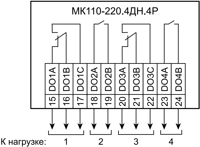
Рисунок 5.3 – Схема подключения к выходу типа электромагнитное реле
